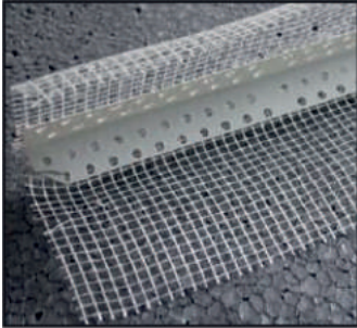
Fileli köşe malzemesi
