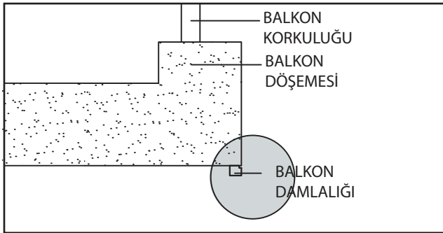
S - 38 FUGALI DAMLALIK PROFİLİ
