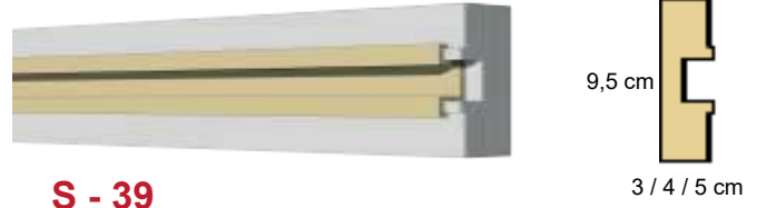
S - 39 DÜZ FUGA PROFİLİ
