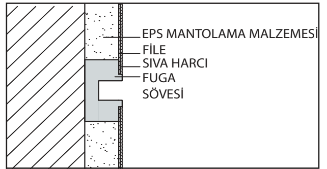
S - 40 TRAPEZ FUGA PROFİLİ
